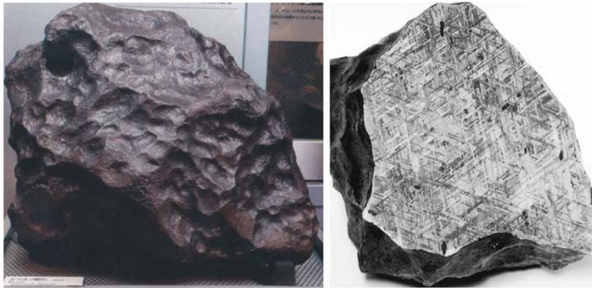
鉄隕石（ギベオン）とウィドマンシュテッテン構造
